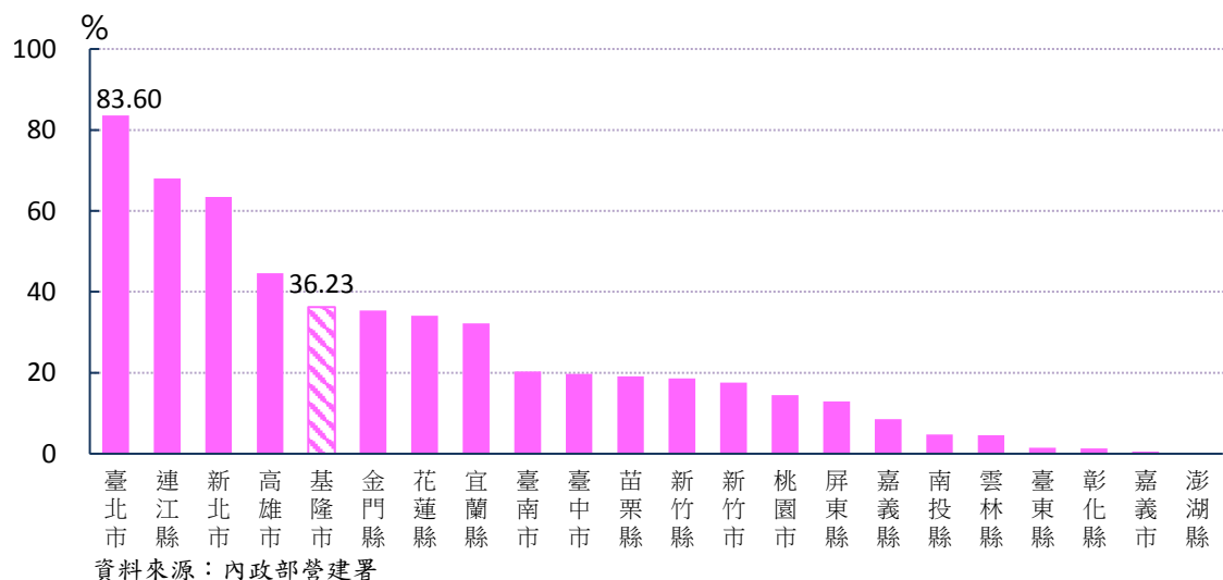
圖 3、108 年底各縣市公共污水下水道普及率
