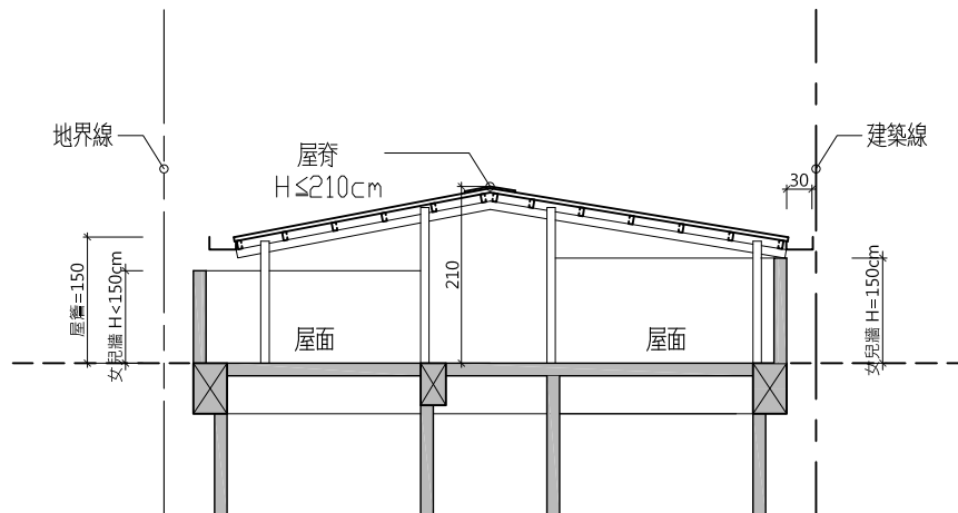
剖面D
