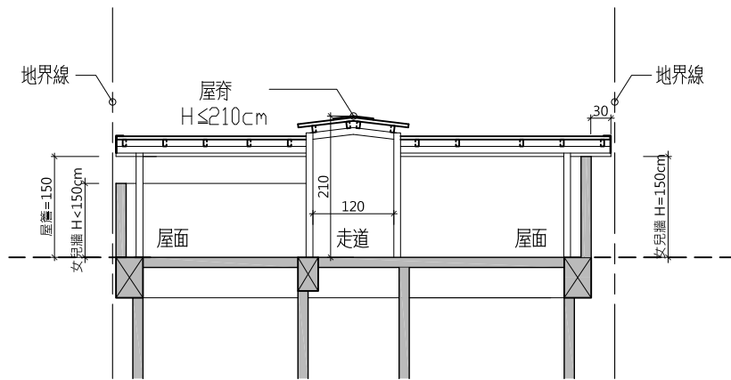
剖面E
