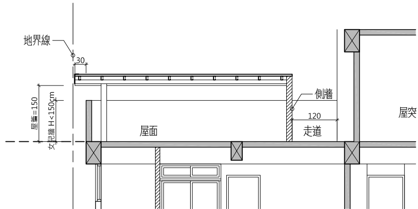
剖面C
