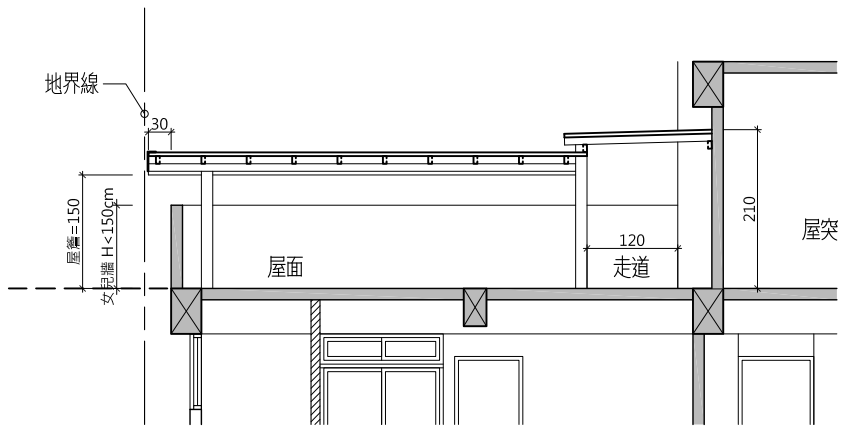
剖面A
