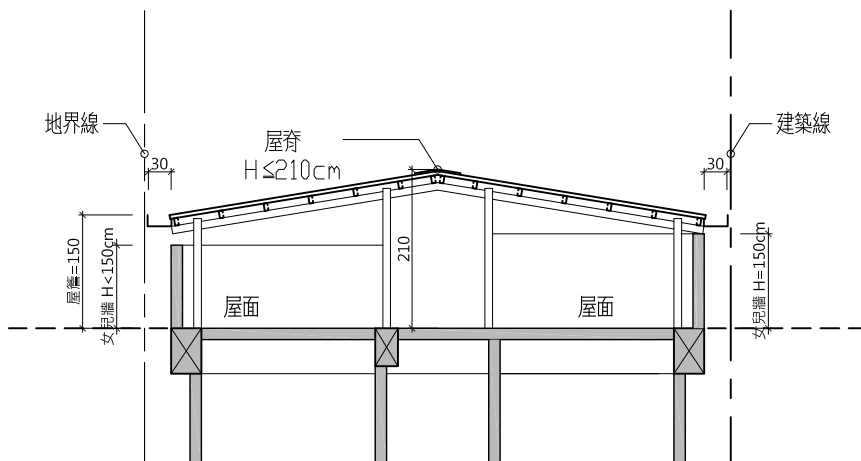
剖面B
