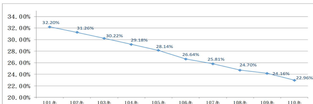
圖 41：基隆地區漏水率下降趨勢圖
