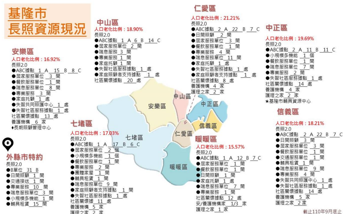
圖 18：基隆市長照資源現況布建地圖
