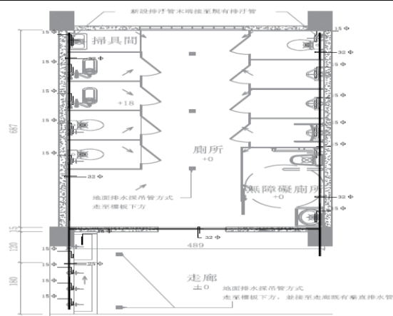
1 A5-3 2樓廁所給水設計平面圖 S:1/100
