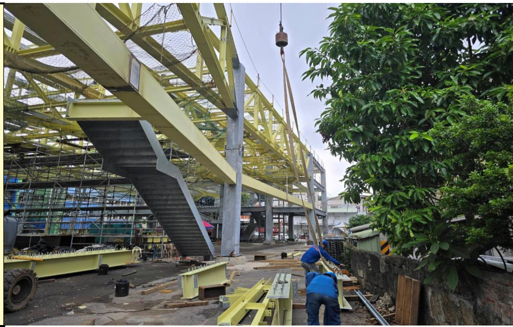
鋼構吊裝
