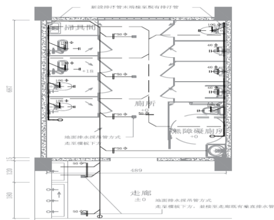
3 A5-3 2樓廁所汙排水設計平面圖 S:1/100
