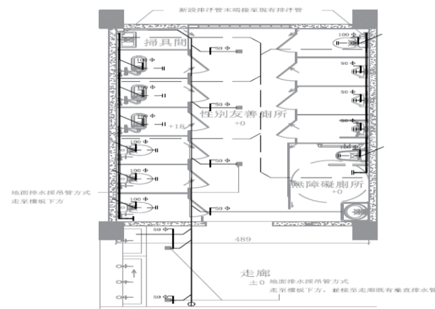
4 A5-3 3樓廁所汙排水設計平面圖 S:1/100
