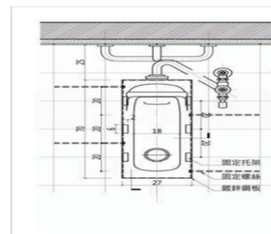
5 A5-3 加長型蹲式便器細部大樣圖 S:1/20
