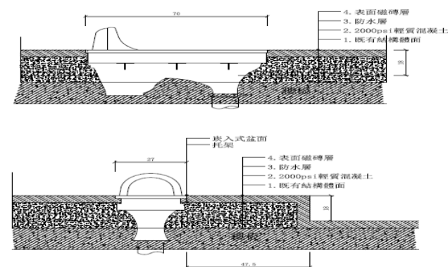
5 A5-3 加長型蹲式便器細部大樣圖 S:1/20
