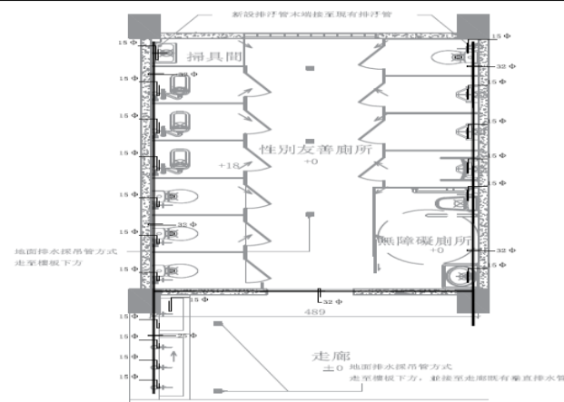
2 A5-3 3樓廁所給水設計平面圖 S:1/100
